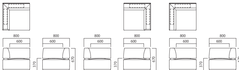
1P 片アーム R (右)
