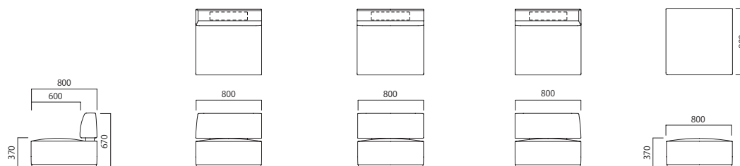
1P アームレス ストレート (中間)
